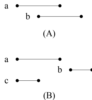
(圖 3) (A) a 與 b 是 overlap；(B) a 與 b 、 c 是 commute。
