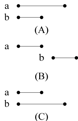
(圖 4) a 與 b 是 commute，則：(A) a 包含 b ；(B) a 與 b 不相交；(C) a 包含於 b 。由 Lemma 3 可知，反轉任一個 Unoriented elementary interval，可得到新的 Oriented elementary intervals，且不會再額外增加 reversal distance (因 cycle 個數不變)。
