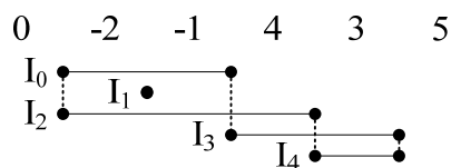
(圖2) I_0, I_1, \dots, I_4 為 P = (0 -2 -1 4 3 5) 的所有 elementary interval。
